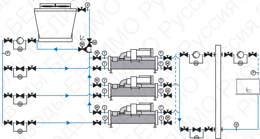
Изоляция чиллеров и байпас градирни
